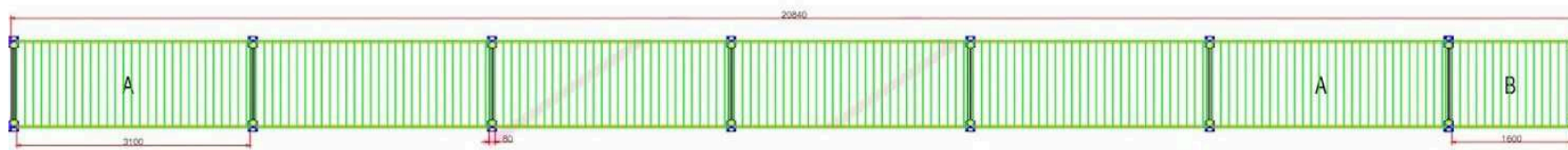
PLANTA BAIXA - ESTRUTURA PORTA PALLET ( PLANO METÁLICO ) ESC. 1:60
