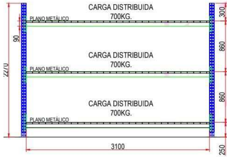
VISTA FRONTAL - MÓDULO A ESC. 1:40
